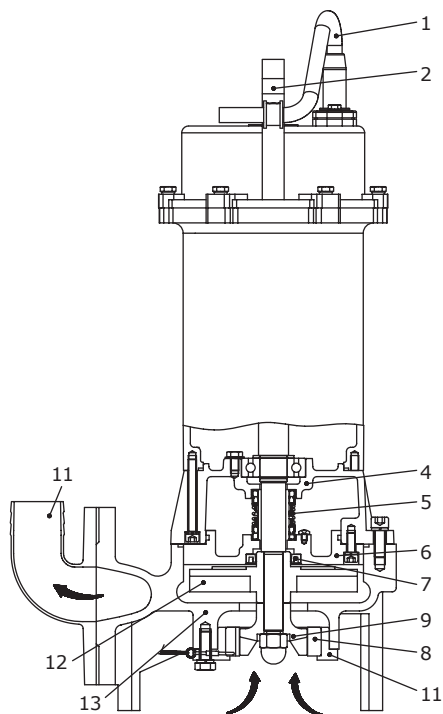
Рис. 1 Насос SG
